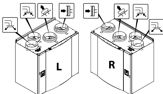
Рис. 3 Соединения воздуховодов
