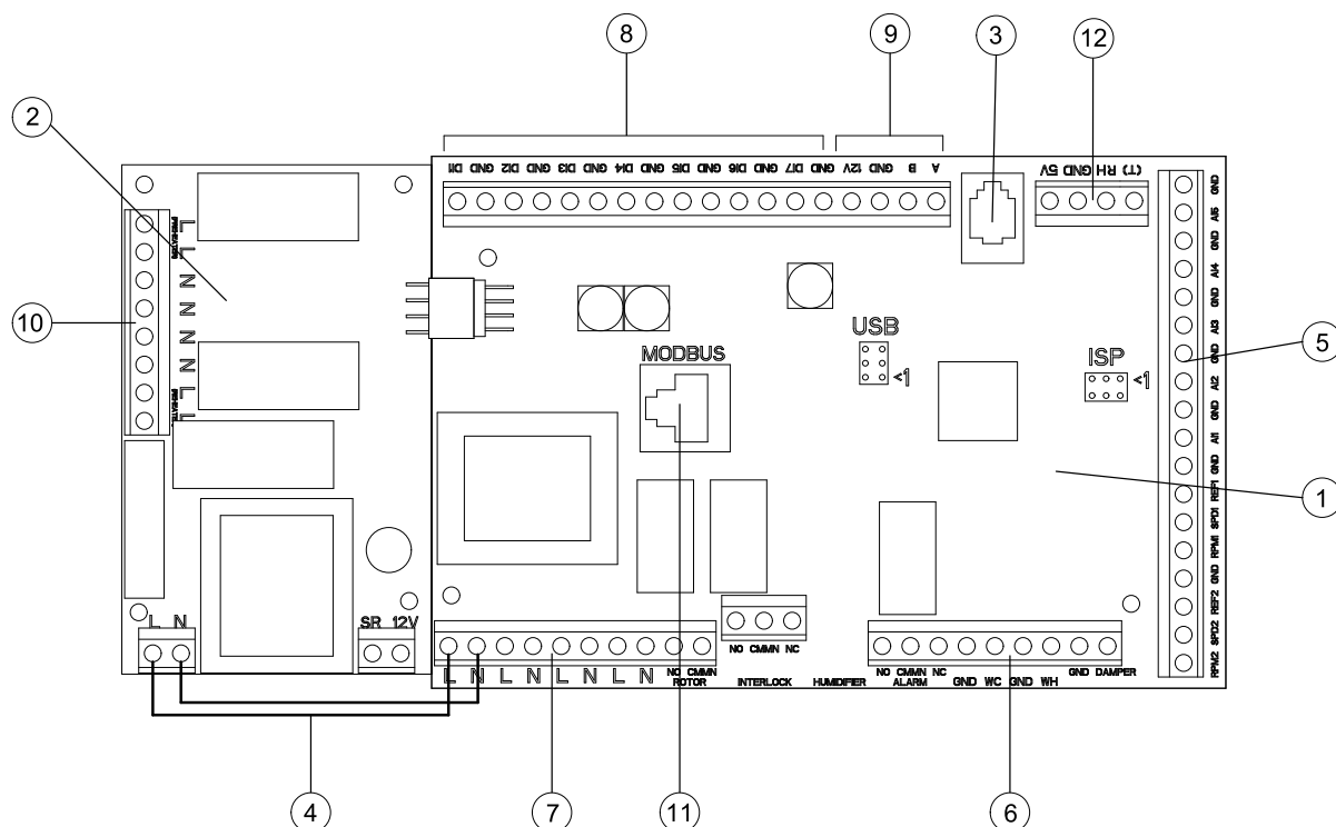
Рис. 9 Печатная плата
