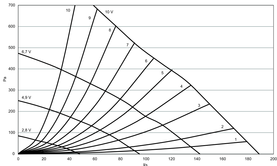
Рис. 7 Фильтр вытяжного воздуха класса G3
