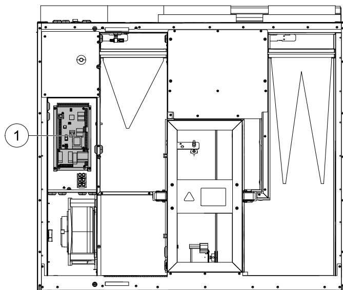
Рис. 8 Местоположение печатной платы
