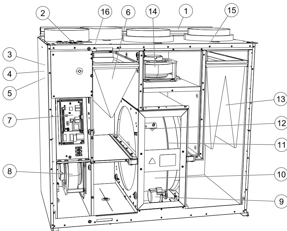
Рис. 11 Внутренние компоненты
