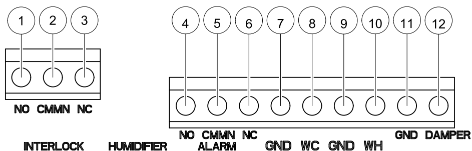
Рис. 10 Контакты платы для подключения внешнего оборудования
